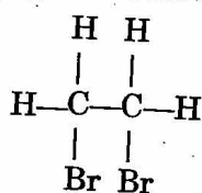
1, 2-dibromoethane
