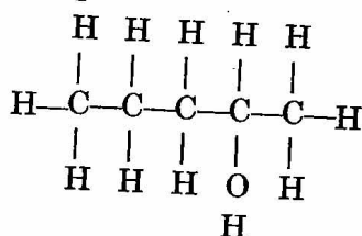
Pentan-2-ol
